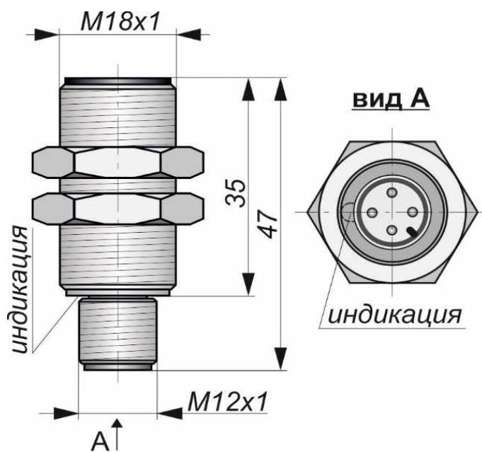
Габаритный чертеж
